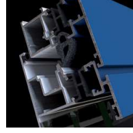
nodo centrale con profili isolatori
